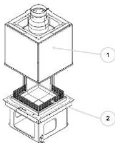
Afb. 68: Bekleding en vuurvaste bakstenen
