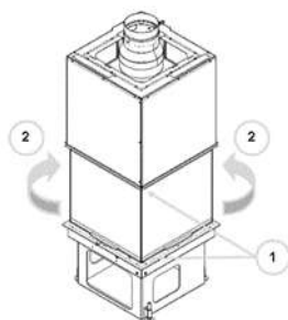
Afb. 65: Draai de deur aan beide kanten open
