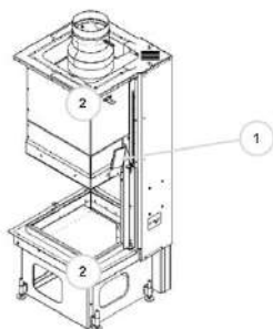
Fig. 69: Unit body
