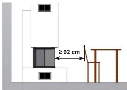
Bild 12: Sicherheitsabstand im Strahlungsbereich
