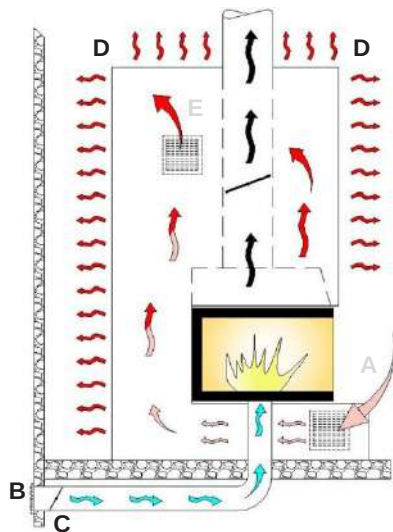
Bild 17: Schnitt durch eine Speicheranlage
