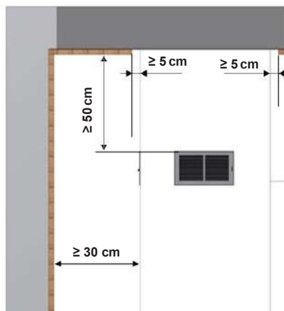
Bild 11: Sicherheitsabstände am Warmluftaustritt
