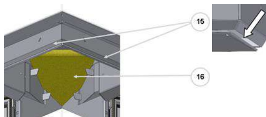
Illustration 5: Déflecteur brise-flammes dans l'avaloir
