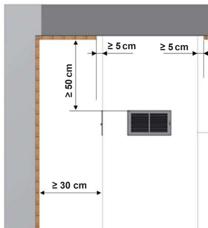
Afb. 11: Veiligheidsafstanden rond opening voor warme lucht
