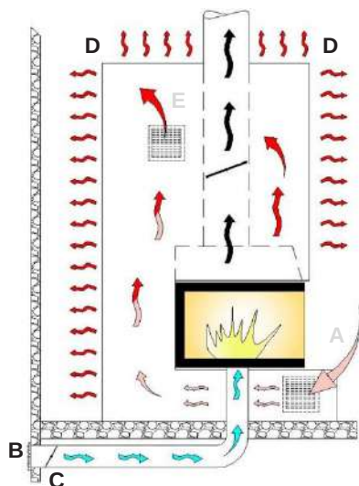
Illustration 17: Coupe à travers un système à accumulation/rayonnement
