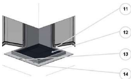
Afb. 4: Overzicht verbrandingskamer
