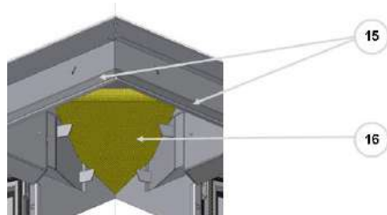
Afb. 5: Stootplaat in rooktrechter
